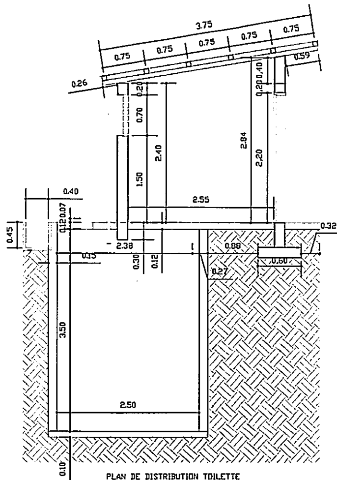
PLAN DE DISTRIBUTION TOILETTE
