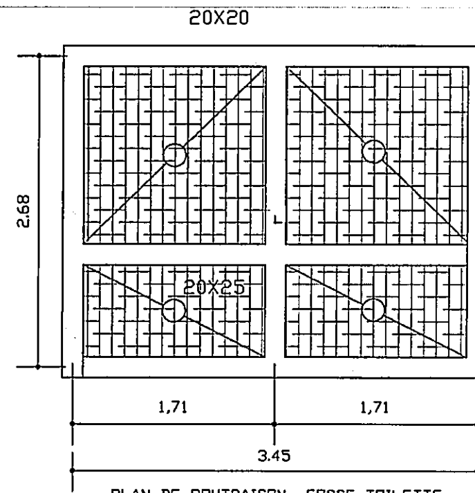
PLAN DE POUTRAISON FOSSE TOILETTE
