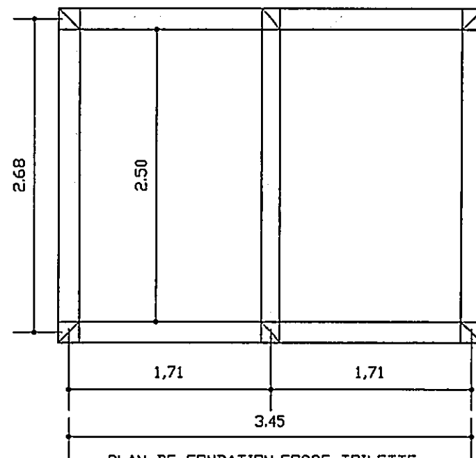
PLAN DE FONDATION FOSSE TOILETTE
